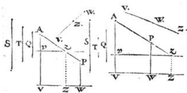
1. Voorval, alwaer het glas en teyckenlick punt elck boven de vloer gegeven sijn.
