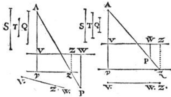
3 Voorval, in 't welck het glas en teyckenlick punt elck beneden de vloer gegeven sijn.
