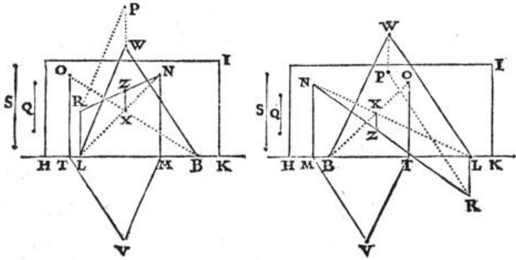
1ste Voorval, alwaer het teyckenlick punt boven de vloer gegeven wort, en het glas tussen 't selve en de voet.
